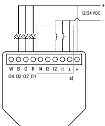
Fig. 2 Wiring in RGBW mode
