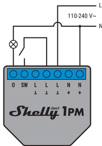
EN Fig. 1. 110-240 V~ Power supply
