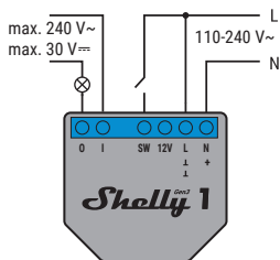
EN Fig. 1. 110-240 V~ power supply
