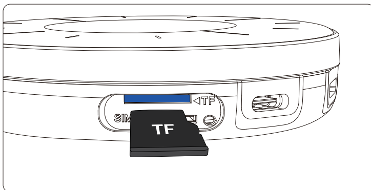
Μέθοδος εγκατάστασης κάρτας TF
