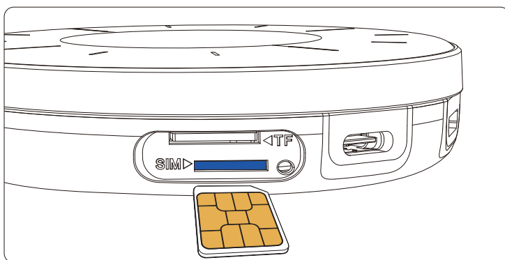
Μέθοδος εγκατάστασης κάρτας Nano SIM
